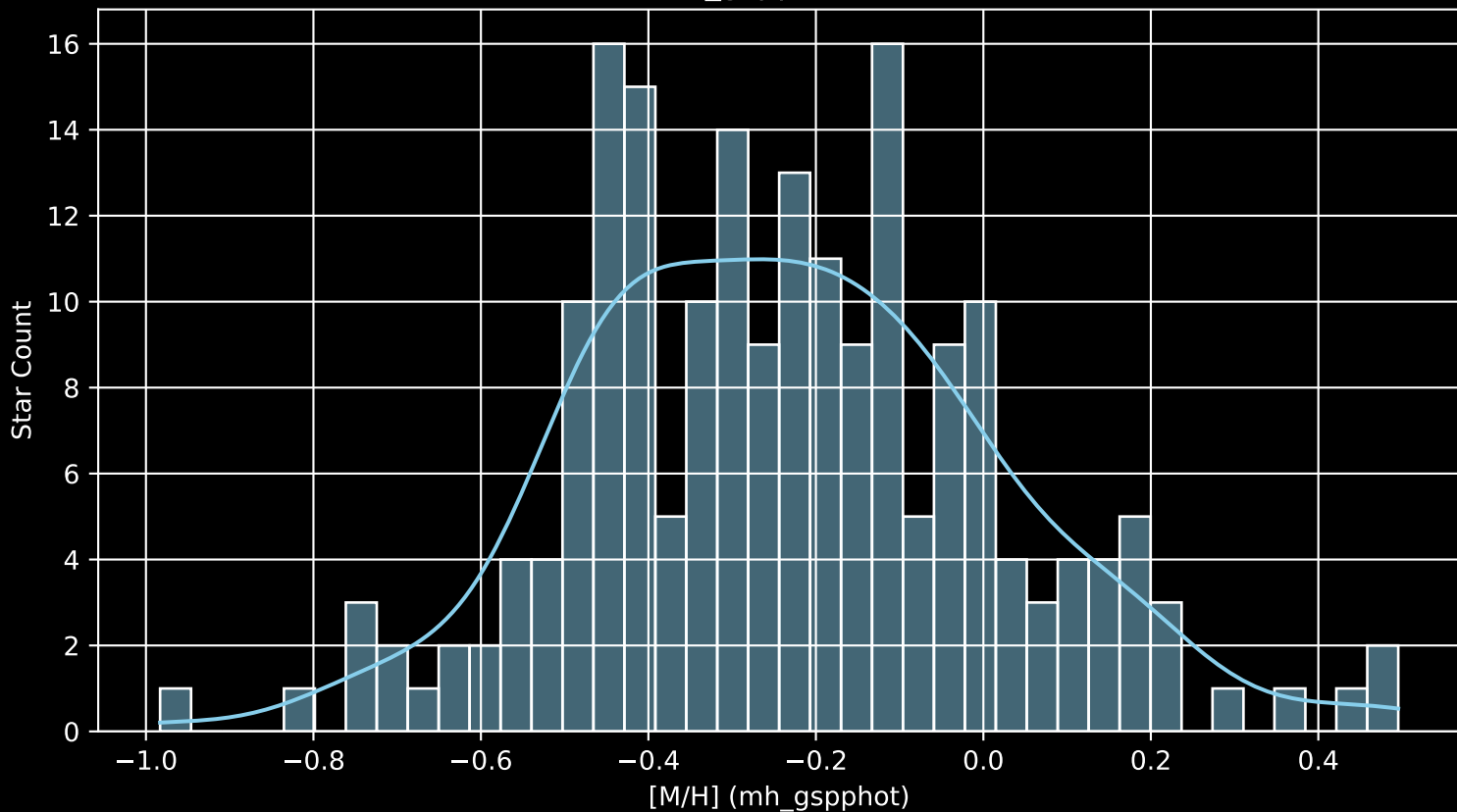
GALAH DR4 Field: [7216] [M/H] (mh_gspphot) (n= 200)
