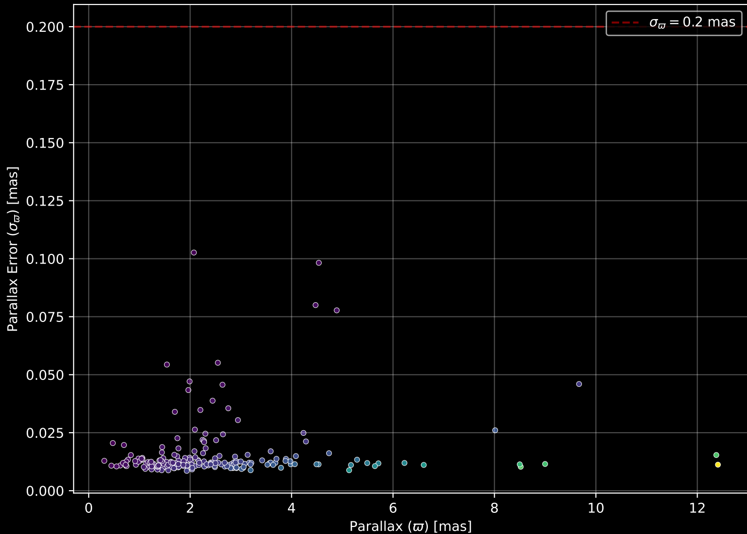
GALAH DR4 Field: [7216] Parallax Quality (n= 200)
