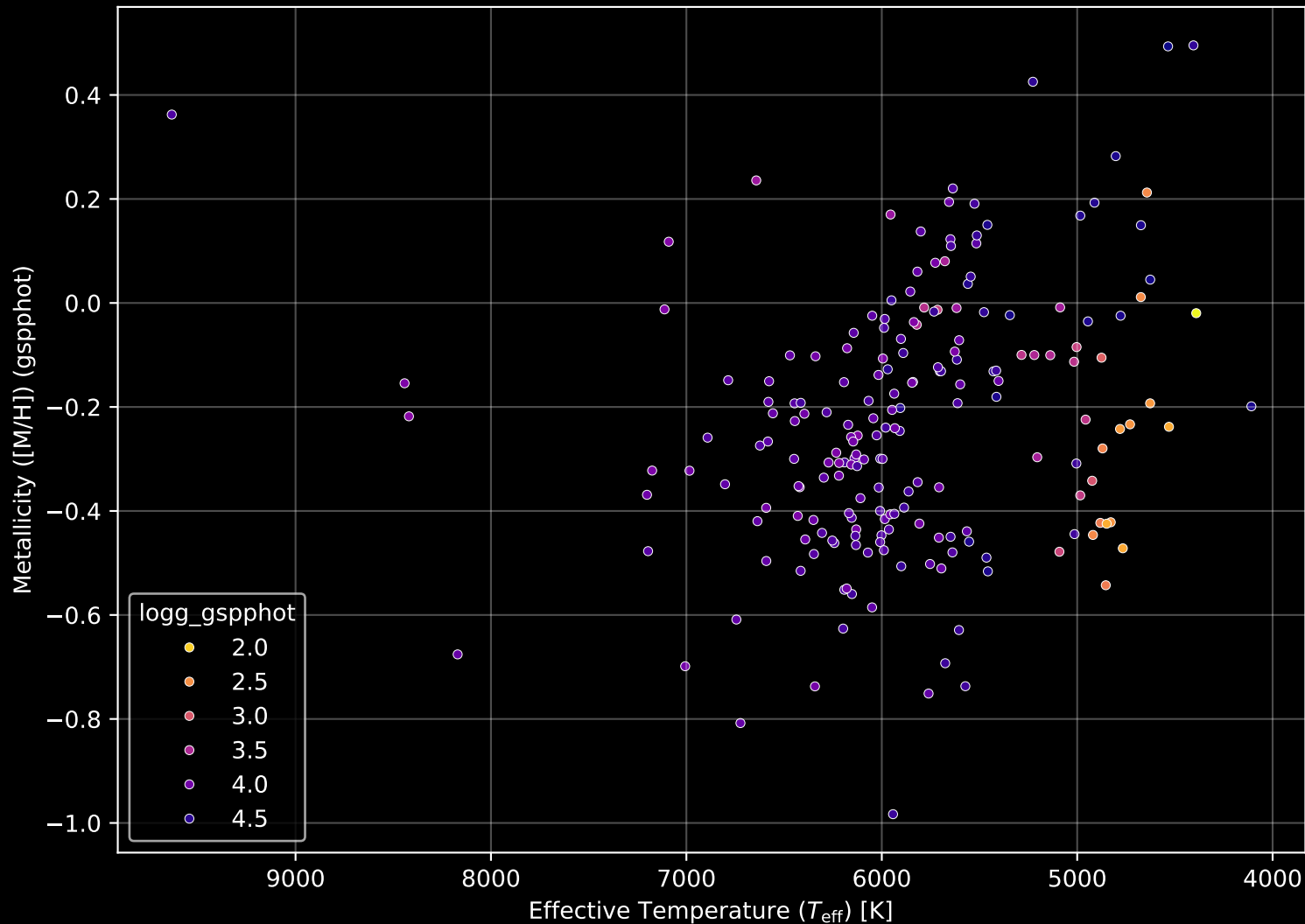
GALAH DR4 Field: [7216] Stellar Population Parameters (n= 200)
