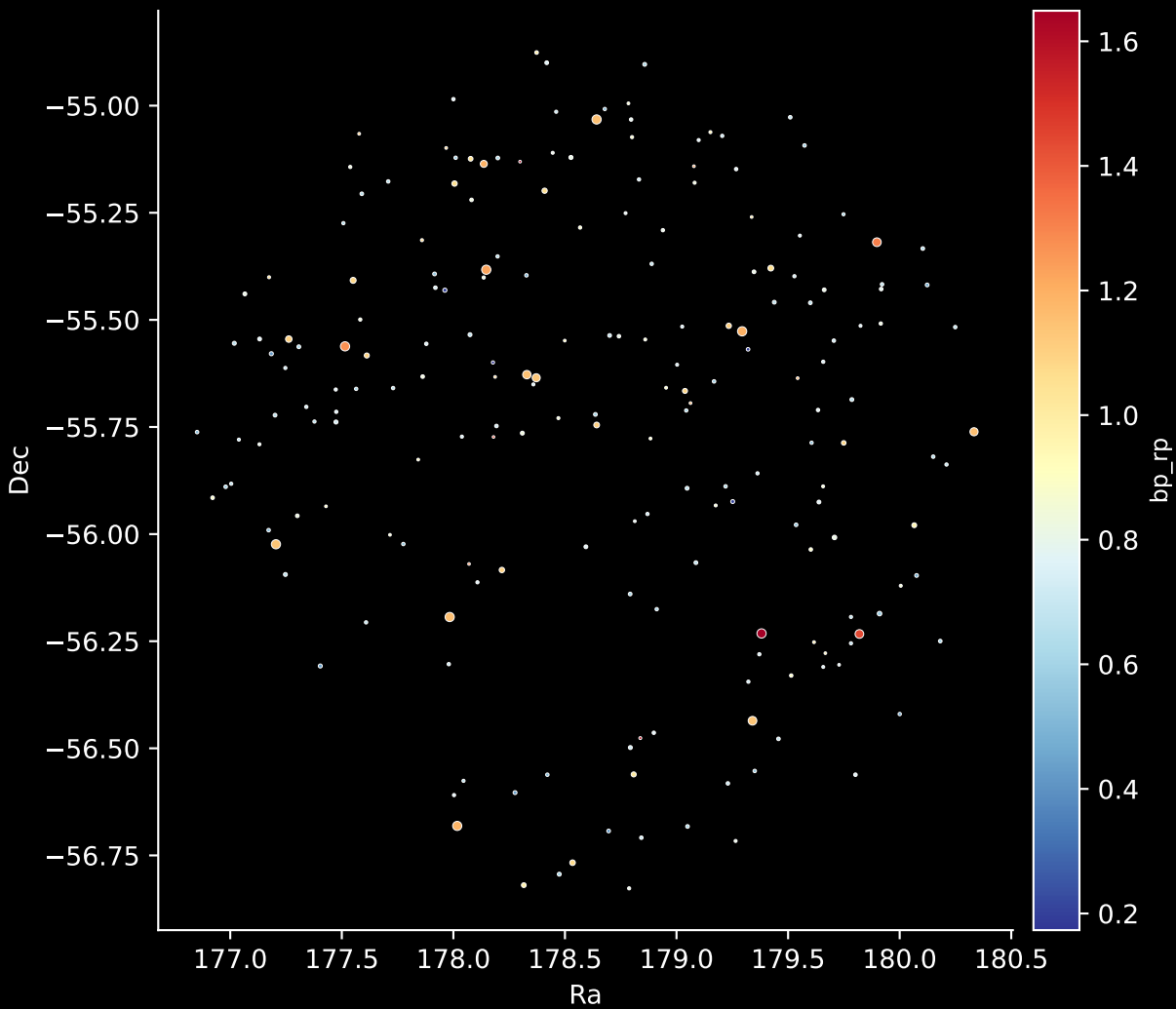
GALAH DR4 Field: [7216] Stars: 200
